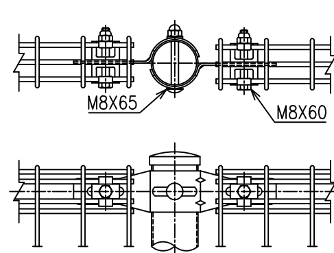
C部詳細図 S=1/4
