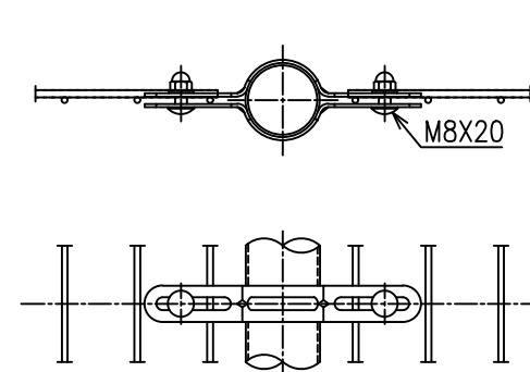
D部詳細図 S=1/4
